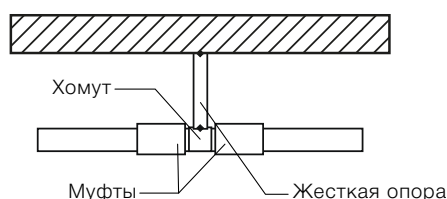
Рисунок 13. Неподвижная опора, выполненная хомутом между муфт
