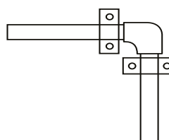
Рисунок 10. Неподвижная опора в местах изгиба
