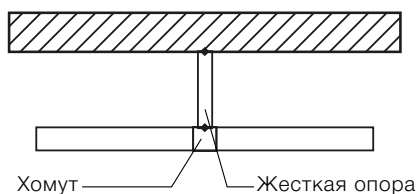
Рисунок 11. Неподвижная опора, выполненная с использованием хомута
