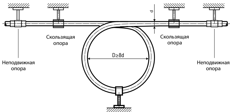
Рисунок 4. Петлеобразный компенсатор
