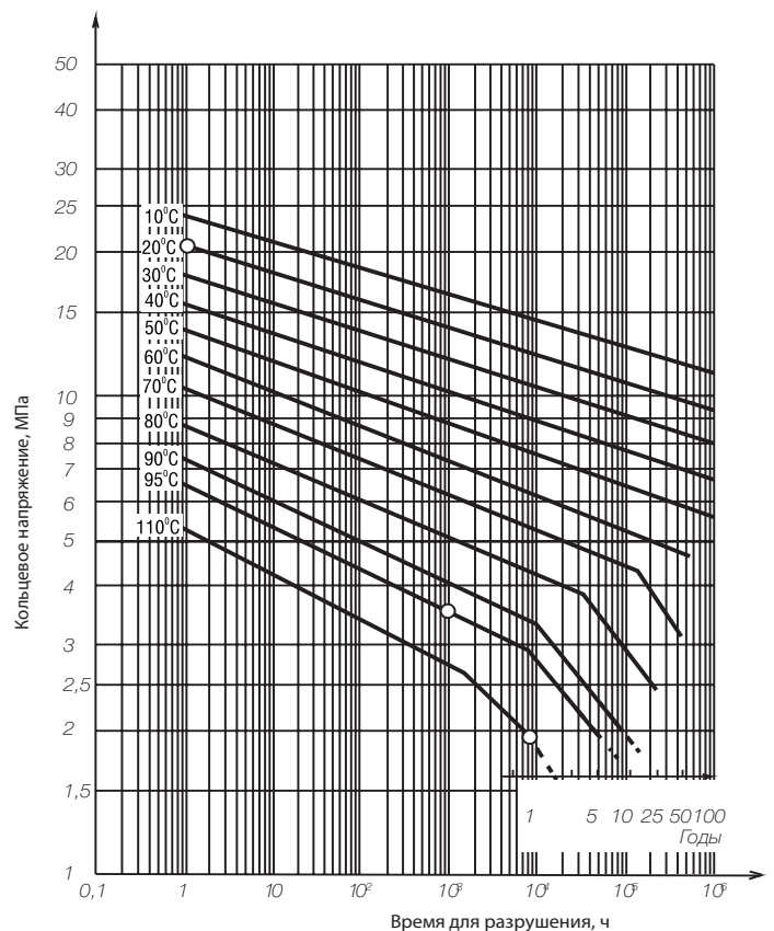
Рисунок 1. Эталонные графики длительной прочности PPR
