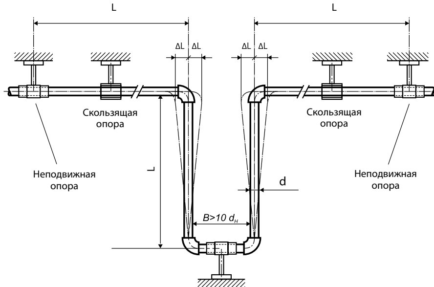
Рисунок 3. П-образный компенсатор
