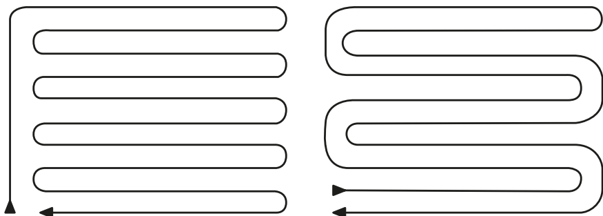
Рисунок 25. Варианты укладки теплого пола змейкой
