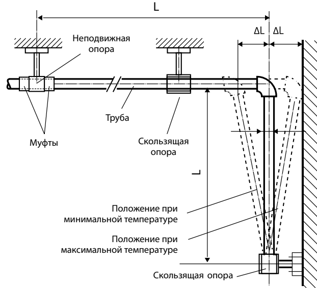
Рисунок 2. Г-образный элемент напорного полипропиленового трубопровода
