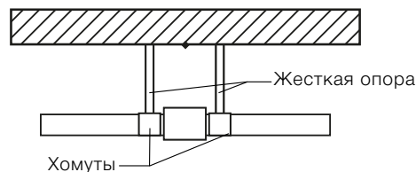
Рисунок 12. Неподвижная опора, выполненная хомутами с двух сторон муфты
