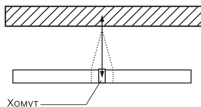
Рисунок 6. Подвижная опора, представленная в виде трех хомутов на подвесе
